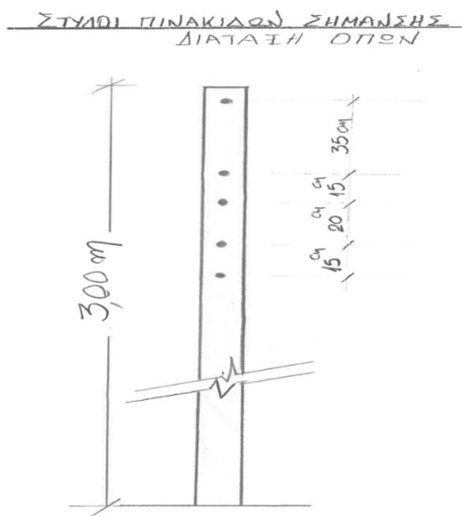
Σχήμα 1 (Διάταξη οπών)
