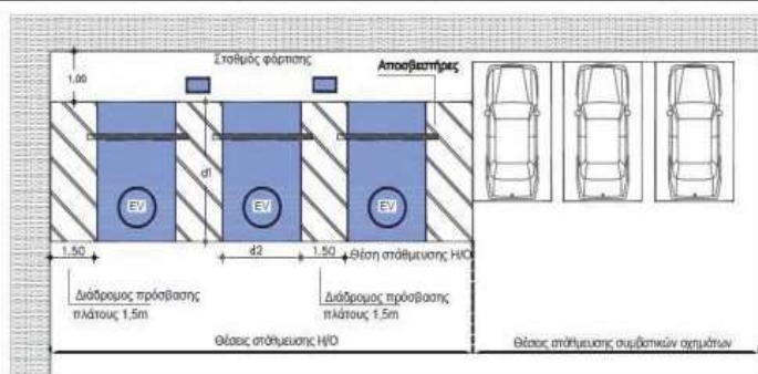
ΣΤΑΘΜΕΥΣΗ ΗΛΕΚΤΡΟΚΙΝΗΤΩΝ ΟΧΗΜΑΤΩΝ ΣΕ ΚΛΕΙΣΤΟ Ή ΥΠΑΙΘΡΙΟ ΧΩΡΟ ΣΤΑΘΜΕΥΣΗΣ
