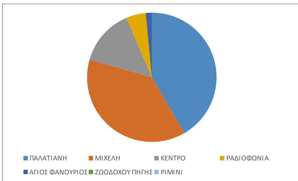
Γράφημα 2: Γεωγραφική κατανομή των διενεργηθέντων ελέγχων μετά το σεισμό της 19/7/2019.
