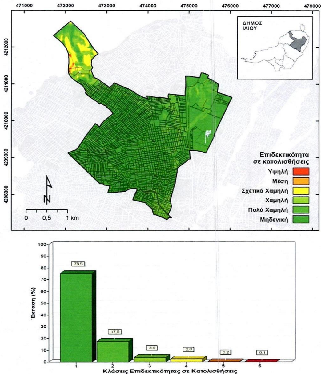
Εικόνα 12: Χάρτης επιδεκτικότητας σε κατολισθήσεις και ιστόγραμμα κατανομής δήμου Ιλίου (Πηγή: Ευθ. Λέκκας et.al., 2010)
