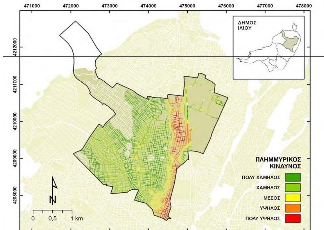
Εικόνα 21: Χάρτης πλημμυρικού κινδύνου του δήμου Ιλίου (Πηγή: Ευθ. Λέκκας et al., 2010)
