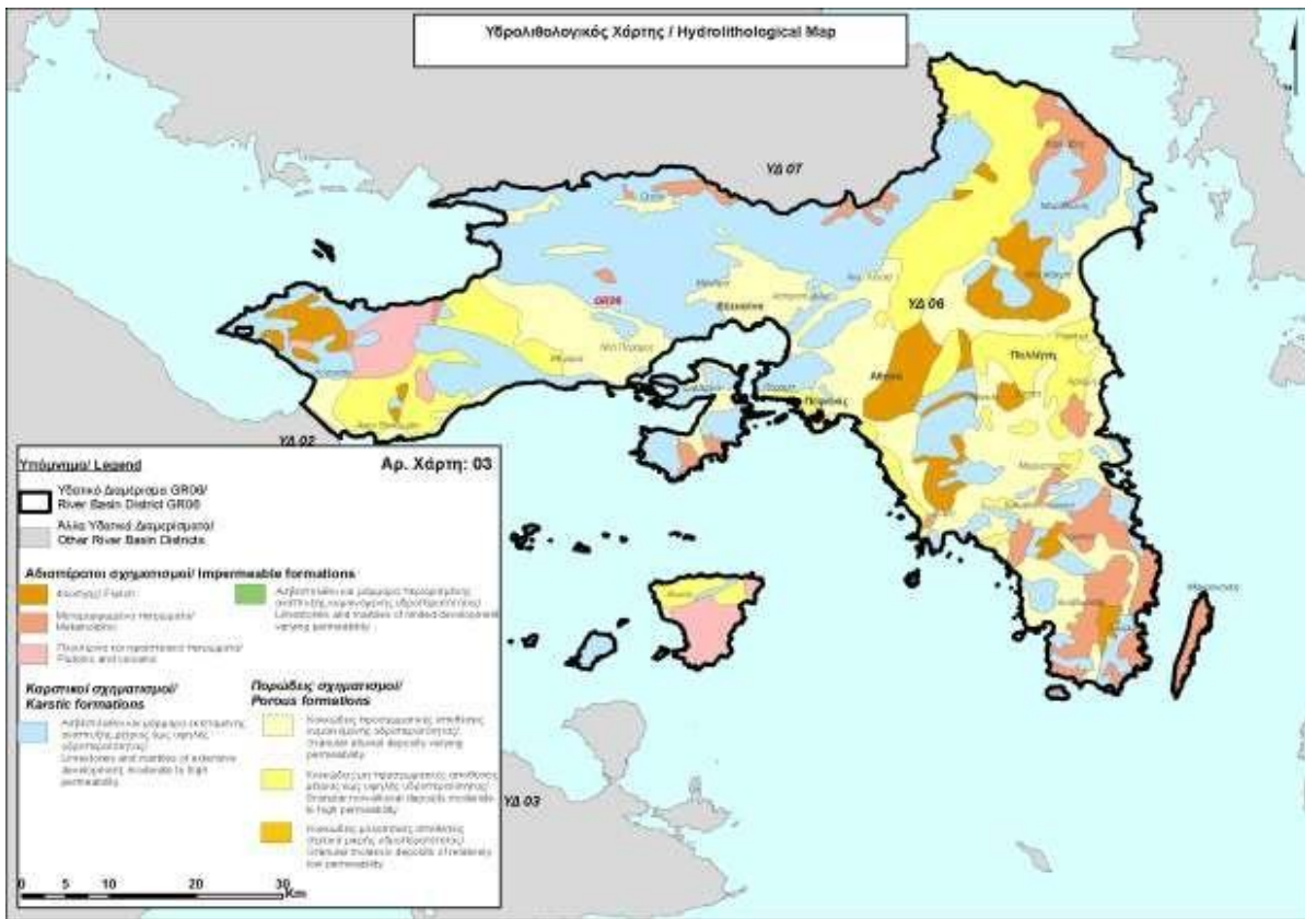
Εικόνα 11: Υδρολιθολογικός χάρτης Υδατικού Διαμερίσματος Αττικής (Πηγή: Υπουργείο Περιβάλλοντος και Ενέργειας/ Ειδική Γραμματεία Υδάτων, 1η Αναθεώρηση Σχεδίου Διαχείρισης των Λεκανών Απορροής Ποταμών του Υδατικού Διαμερίσματος Αττικής (ΕΛ06), Μάιος 2017)
