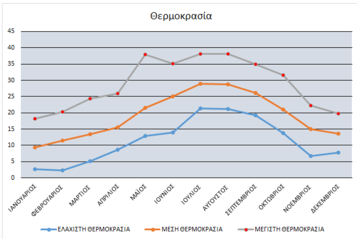
Διάγραμμα 7: Διακύμανση μέσων, μέγιστων και ελάχιστων θερμοκρασιών (Πηγή: ίδια επεξεργασία στοιχείων Μετεωρολογικού Σταθμού Ιλίου)
