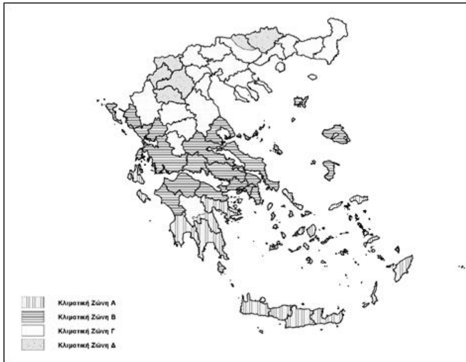
Εικόνα 5: Σχηματική απεικόνιση των κλιματικών ζωνών της ελληνικής επικράτειας (ΦΕΚ 2367/Β'/12-7-2017)
