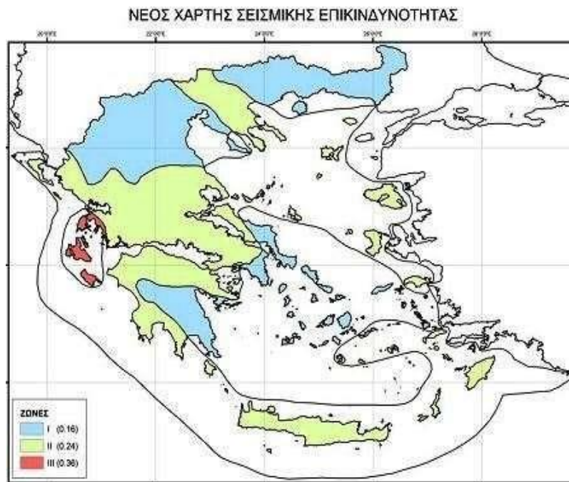
Εικόνα 13: Νέος χάρτης σεισμικής επικινδυνότητας
