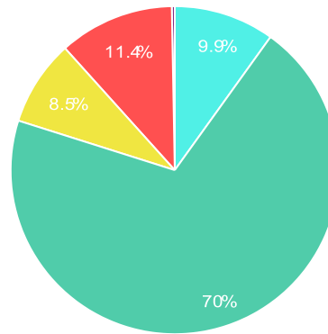
Γράφημα 3: Ποιότητα ατμόσφαιρας-Σταθμός μέτρησης Περιστερίου-21/10/2019-21/10/2010 (Πηγή: www.eea.europa.eu/data-and-maps/data/airreporting-2 )
