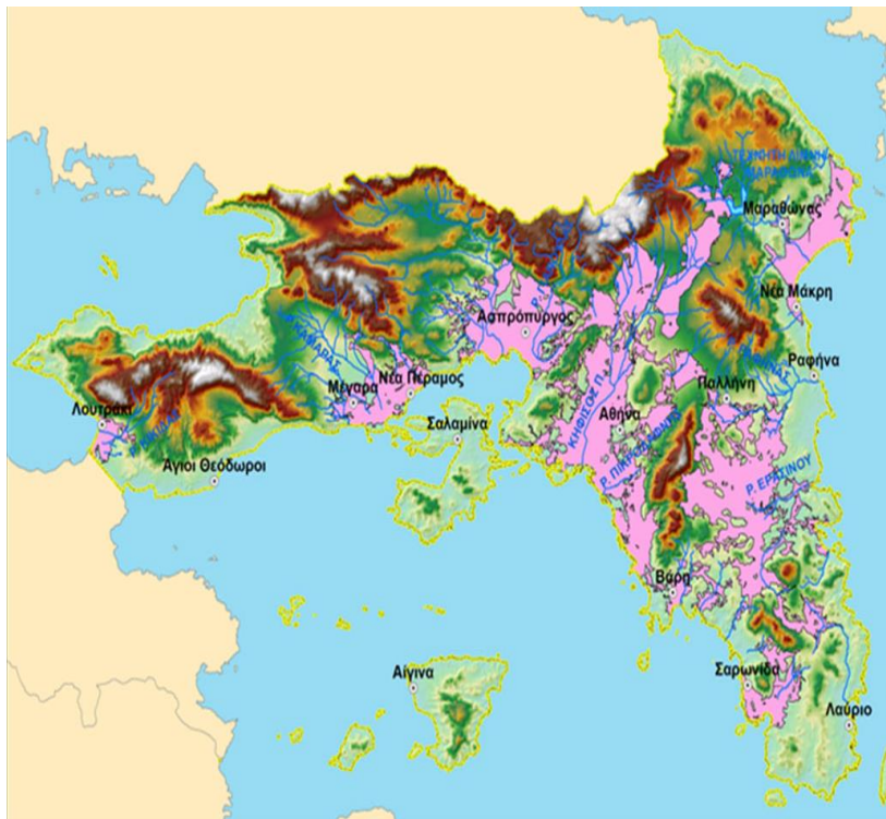
Εικόνα 20: Ζώνες δυνητικά υψηλού κινδύνου πλημμύρας στο ΥΔ Αττικής (ΦΕΚ 2693/Β'/6-7-2018)
