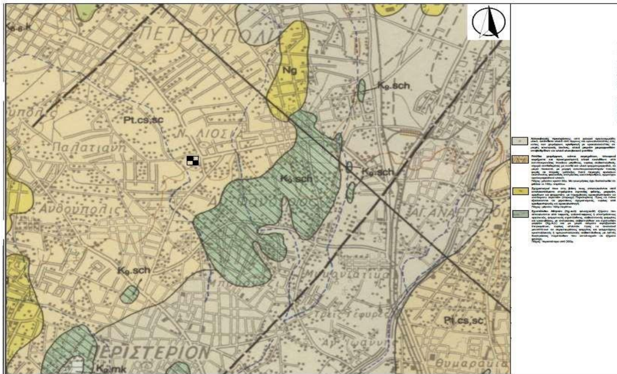
Εικόνα 8: Γεωλογικός χάρτης (IGME 1986)
