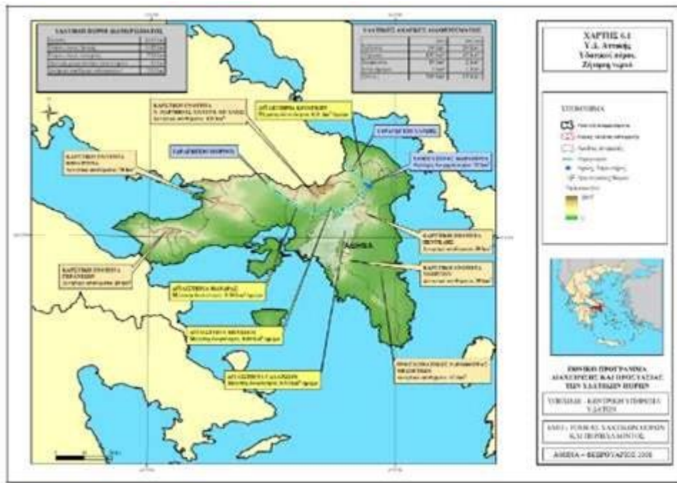
Εικόνα 9: Υδατικό διαμέρισμα Αττικής
