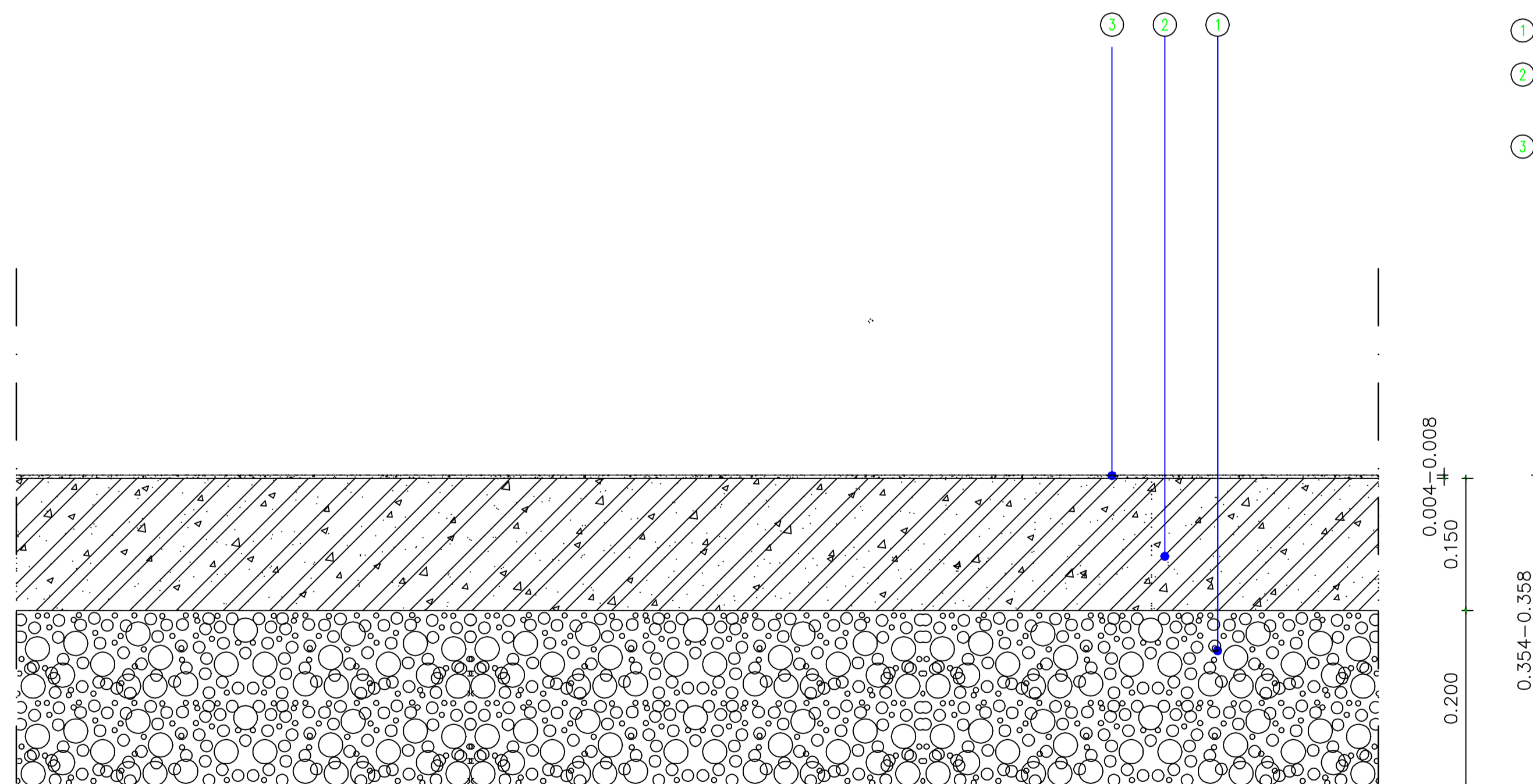
ΛΕΠΤΟΜΕΡΕΙΑ ΔΑΠΕΔΟΥ ΠΛΑΤΕΙΑΣ ΧΑΛΑΖΙΑΚΟ
