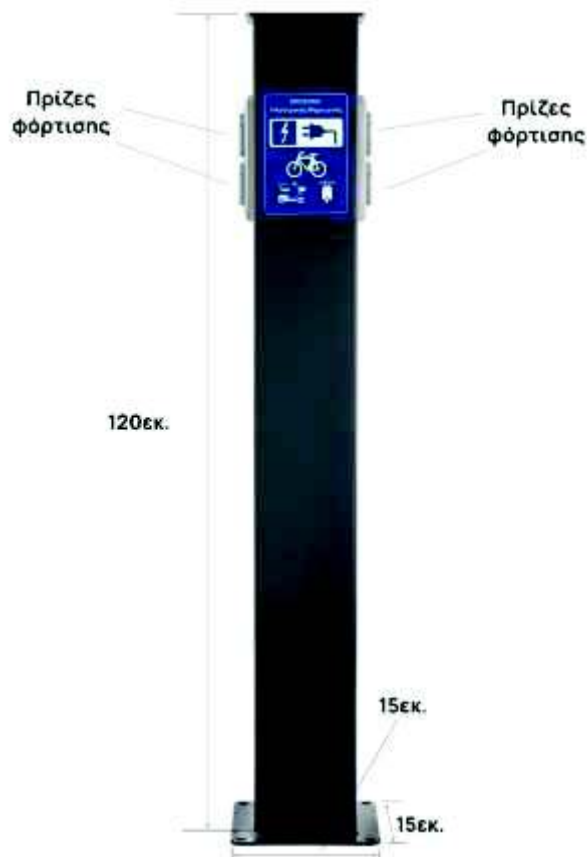
Ενδεικτικό σχέδιο του Σταθμού Φόρτισης
