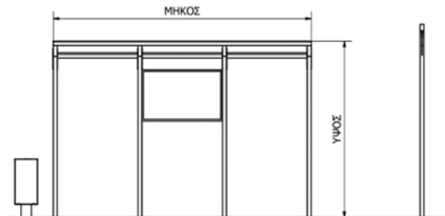
Εικόνα 3 : Ενδεικτικά σκαριφήματα όψης, κάτοψης τύπου Γ
