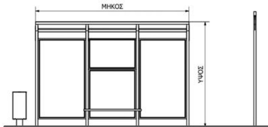
Εικόνα 2 : Ενδεικτικά σκαριφήματα όψης, κάτοψης τύπου Β
