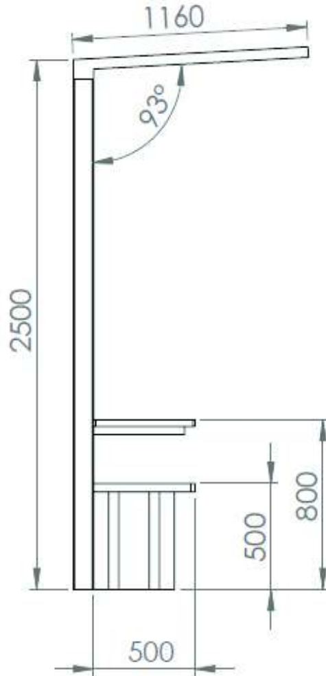
Ενδεικτικό 2D σχέδιο
