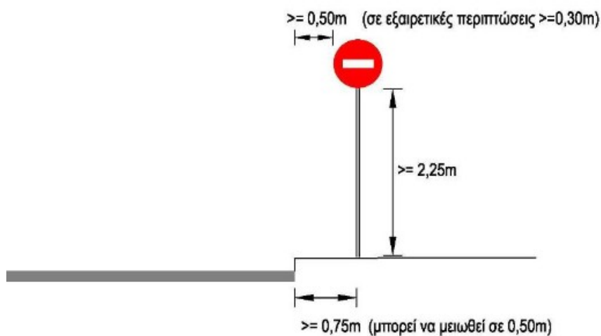
Εικόνα 2: Τοποθέτηση κατακόρυφης σήμανσης σε αστική οδό με πεζοδρόμιο
