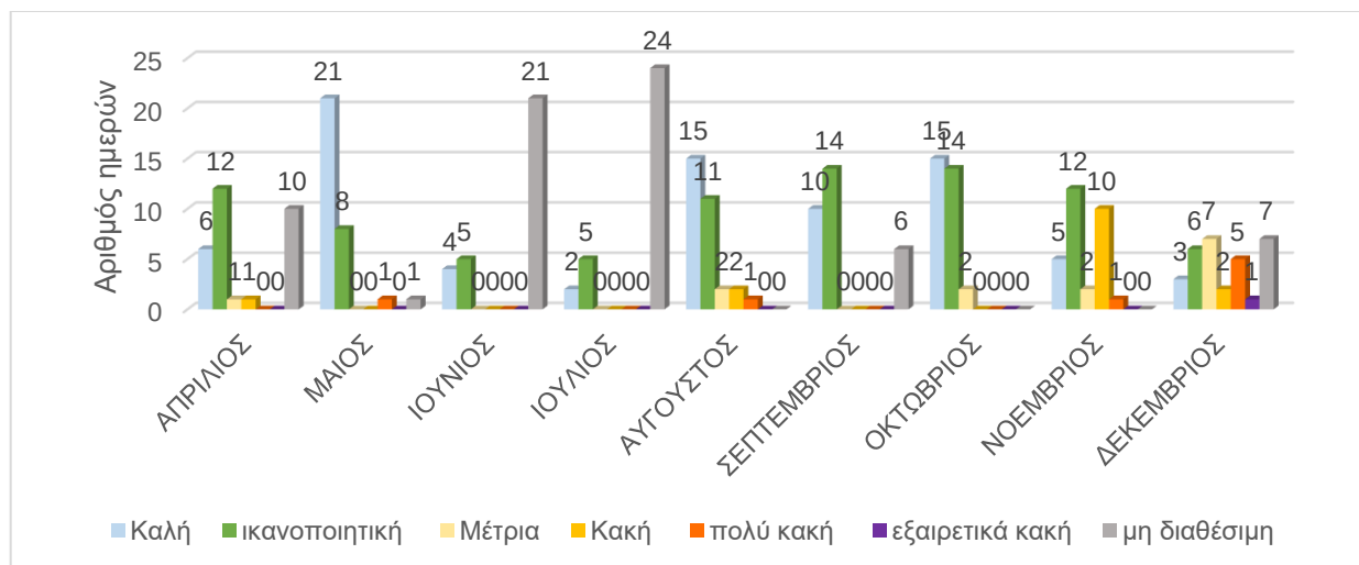
Διάγραμμα 38: Ποιότητα της ατμόσφαιρας στο Δήμο Ιλίου το έτος 2021 ως προς την εξέταση του ρύπου PM 2,5
