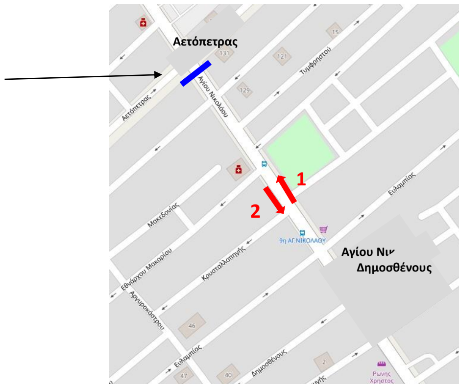
Εικόνα 1.2: Τοποθέτηση καταγραφικών μηχανημάτων επί της Αγίου Νικολάου
