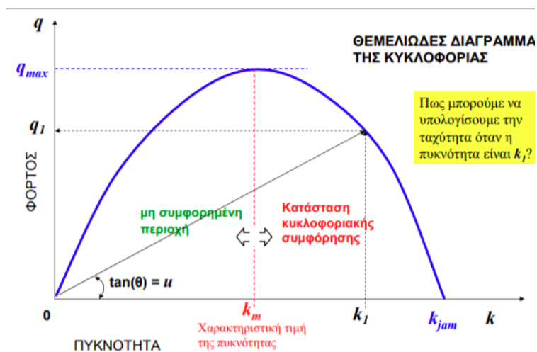
Εικόνα 1.3: Διάγραμμα φόρτου- πυκνότητας
